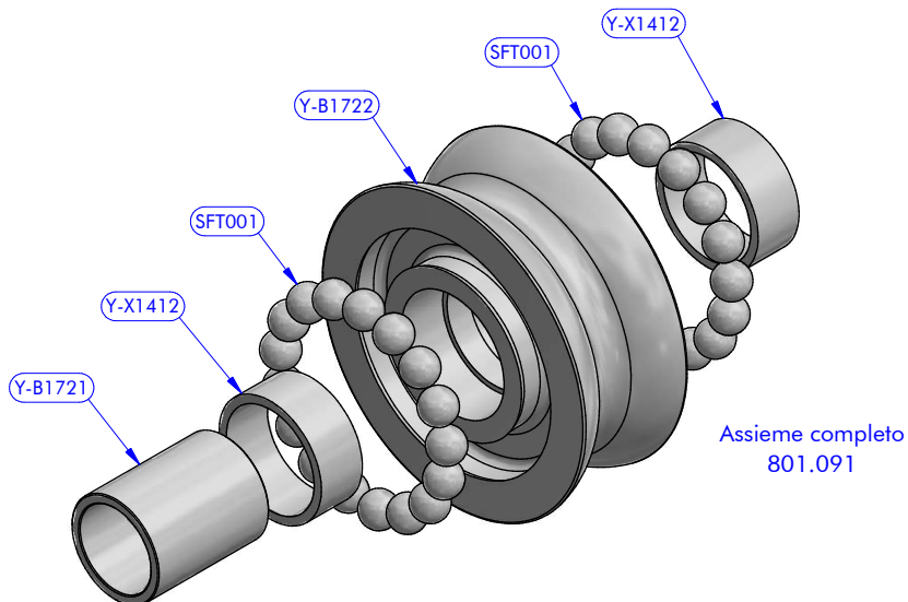
ELENCO PARTI 801.091
